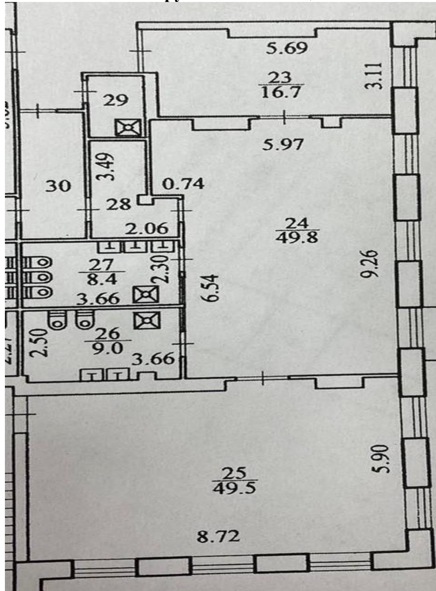
Схема группового помещения
